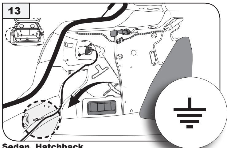
E-Satz Stecker e-kit socket
