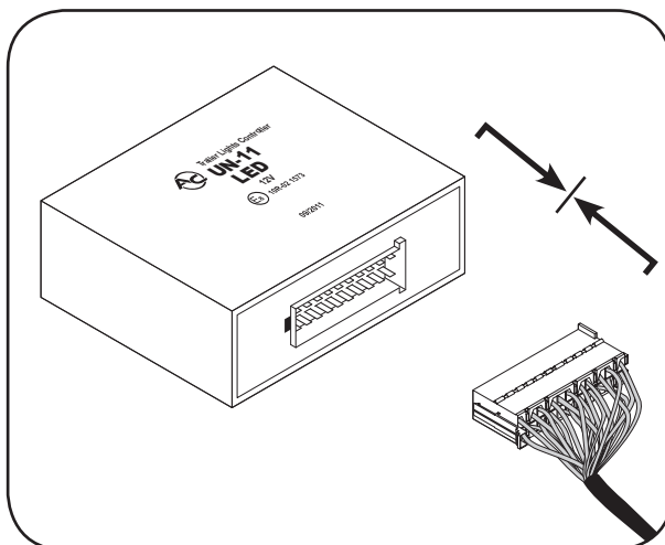
Modul UN-11 → Stecker 22 pin E-Satz modul UN-11 → socket 22 pin e-kit
