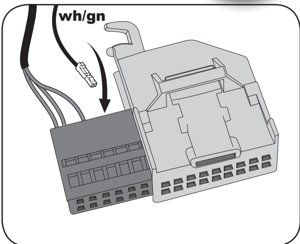
E-Satz wh/gn → PIN 8 e-kit wh/gn → PIN 8
