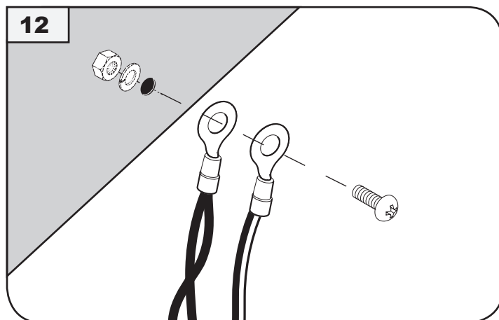
E-Satz 2x bn → , + wh/bn 13 pin e-kit 2x bn → , + wh/bn 13 pin
