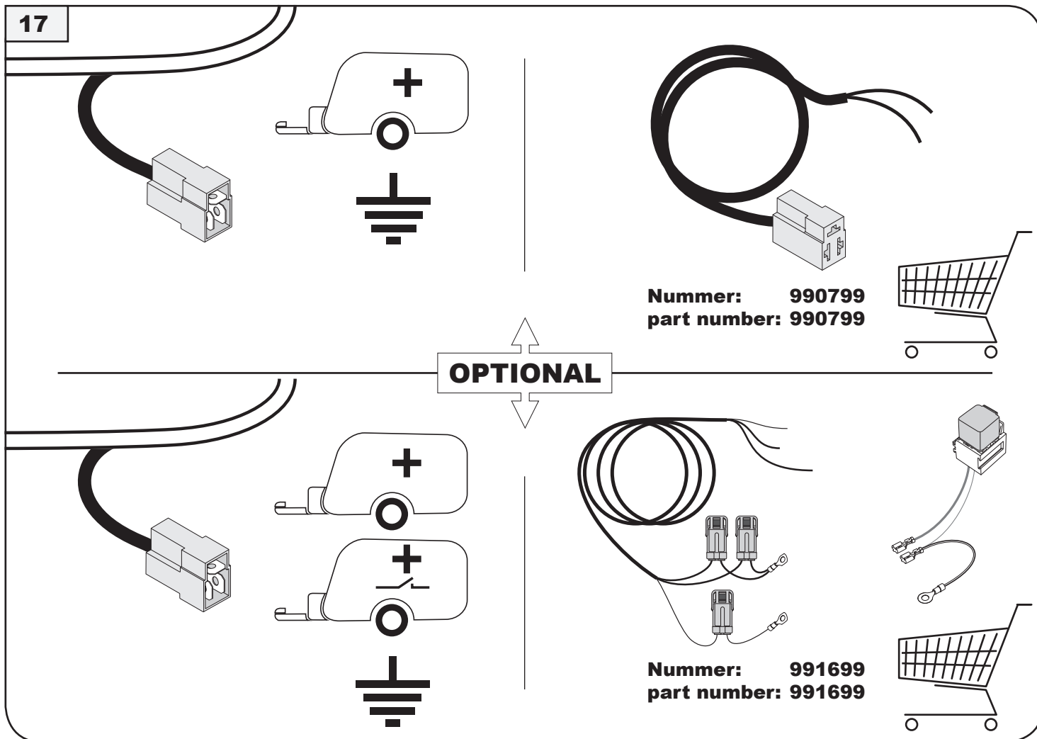
Sicherung 15A → fuse 15A →
