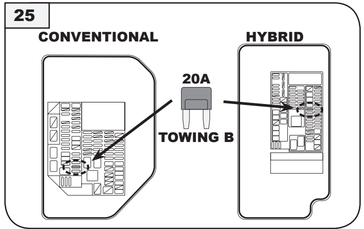
Sicherung 20A → TOWING B fuse 20A → TOWING B
